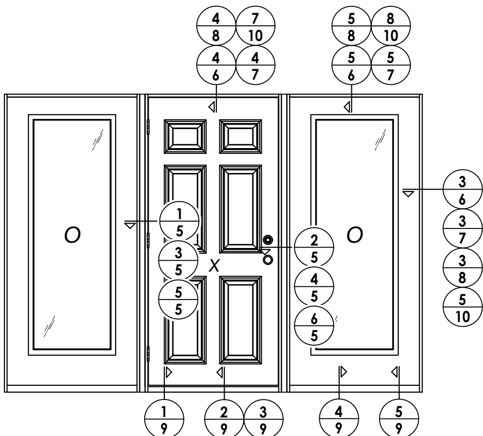
ELEVATION OXO
